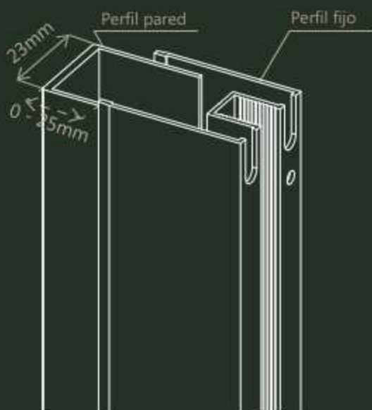
Perfil laterales expansor fijo
