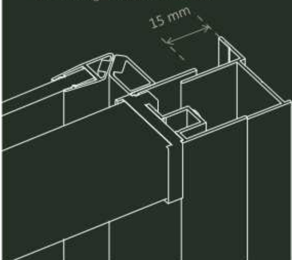
Perfil fijo
