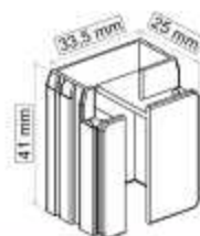
Conector inferior 300 izquierda ABS REF: 019601 10 € REF: 019602 10 €
