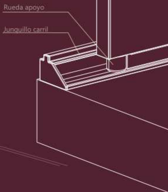
Deslizamiento puerta
