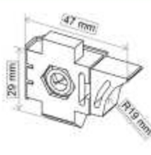
Freno Conjunto REF: 013601 20 €
