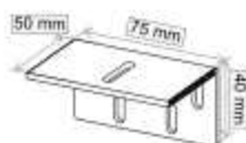
Sujeción a pared REF: 031401 50 € REF: 031402 50 € Acero
