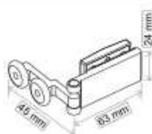
Rodamiento superior Acero REF: 023101 50 € REF: 023102 50 €
