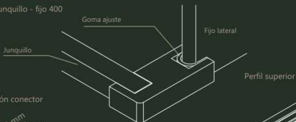
Perfil superior clipado
