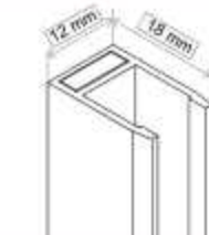
Perfil imán pack R Aluminio REF: 001601 30 € REF: 001602 35 €
