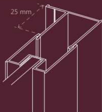
Tapa perfil lateral superior
