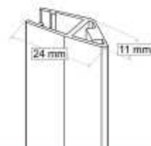
Goma magnética
