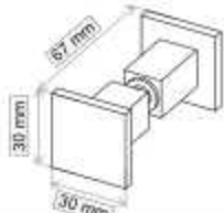
Tirador REF: 024801 50 €
