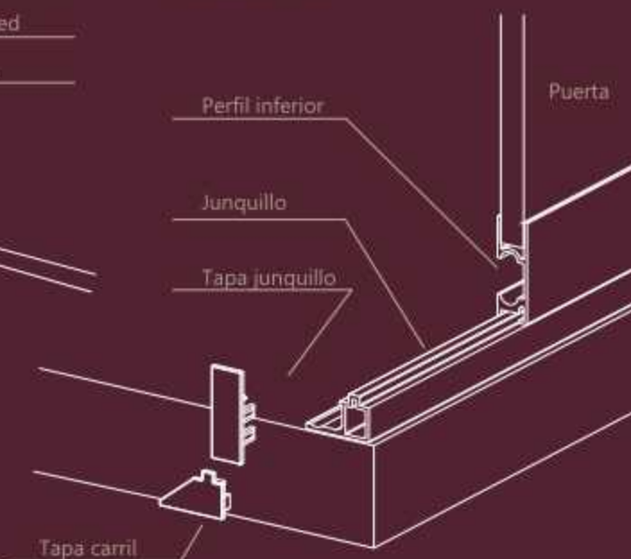
Junquillo 100F
