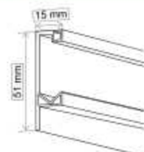
Perfil superior Acero REF: 013501 154 €
