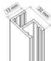
Perfil fijo - fijo Aluminio REF: 006801 70 € REF: 006802 80 €
