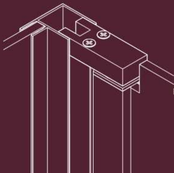
Junquillo
