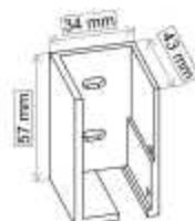
Conector izquierda REF: 017601 45 €
