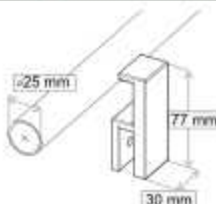
Perfil superior con pinza Acero REF: 013701 139 €
