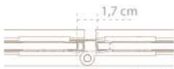
Espacio entre cristales.
