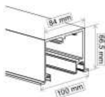
Perfil superior Aluminio. REF: 022008 ● 160 €
