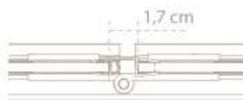
Espacio entre cristales.
