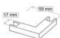
Ángulo unión junquillos Acero REF: 039601 20 €
