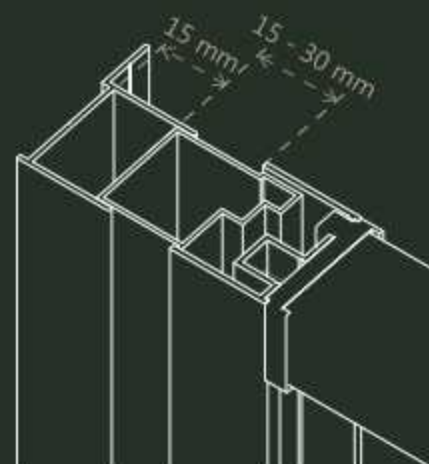
Expansión perfil opcional
