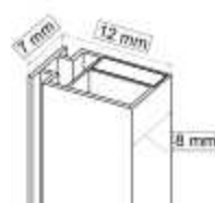
Goma magnética para perfil Goma REF: 032500 25 € REF: 032502 25 €
