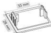
Tapa perfil lateral REF: 005501 10 €
