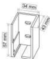
Conector derecha REF: 017701 45 €
