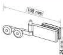
Rodamiento inferior Acero REF: 023201 50 € REF: 023202 50 €
