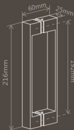
Tirador
