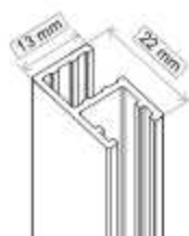
Perfil fijo + fijo 90° Aluminio REF: 006801 50 €
