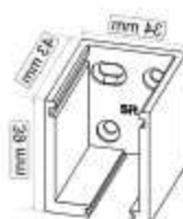
Conector izquierda Acero REF: 020001 25 € REF: 020002 30 €
