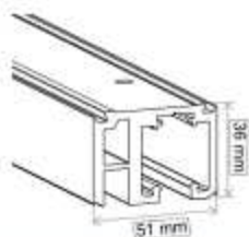
Perfil superior con fijo Aluminio REF: 021601 60 €
