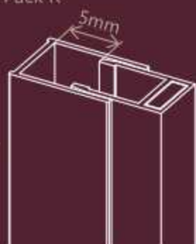
Expansión Pack R
