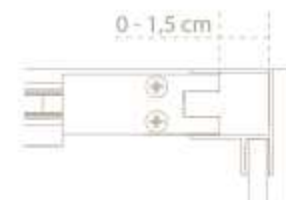
Expansión pack de giro + perfil C.
