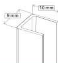
Perfil pared magnético Acero REF: 002301 31 €
