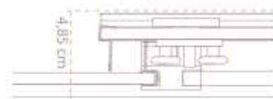
Retranqueo puerta.
