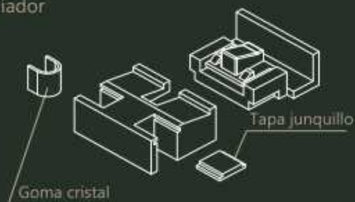
Guiador
