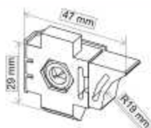
Freno REF: 013601 20 € Conjunto
