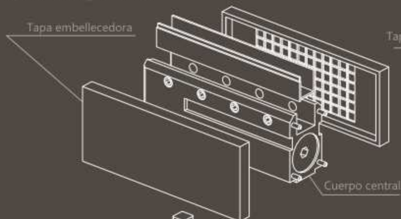
Explosión bisagra inferior.
