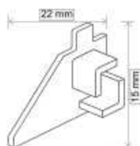
Tapa Junquillo 100F derecha ABS REF: 040901 10 € REF: 040902 10 €
