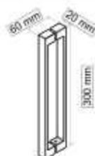
Tirador REF: 023701 55 € Acero
