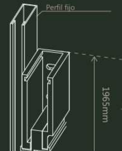
Perfil 300 T
