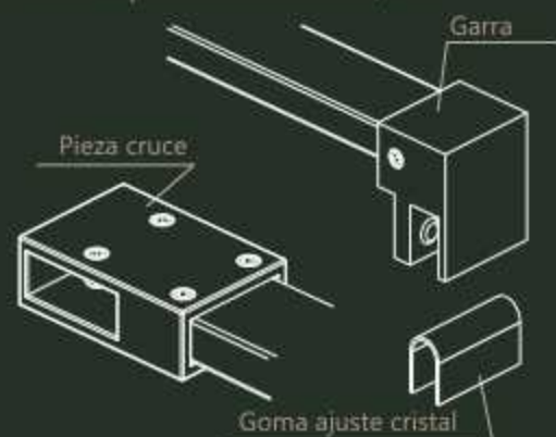
Tensor opcional lateral 400, 800
