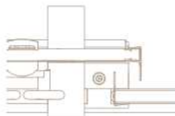
Cierre con goma de cruce.
