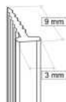
Goma de presión Goma. REF: 033400 11 €
