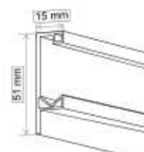
Perfil superior REF: 013201 154 € Acero
