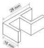
Pieza de conexión cristal fijo nº 5 REF. 039801 10 € REF. 039802 Acero 10 € REF. 039803 10 € REF. 039804 10 € REF. 039805 10 € REF. 039806 10 €
