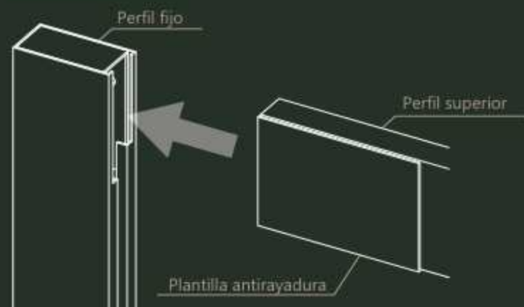
Plantilla antirayadura
