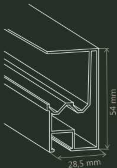
Esquema perfil superior
