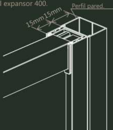
Perfil expansor 400.
