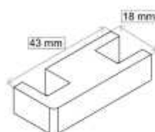
Unión angular junquillo 400 Acero REF: 040401 10 € REF: 040402 12 €
