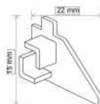
Tapa Junquillo 100F izquierda ABS REF: 041001 10 € REF: 041002 10 €
