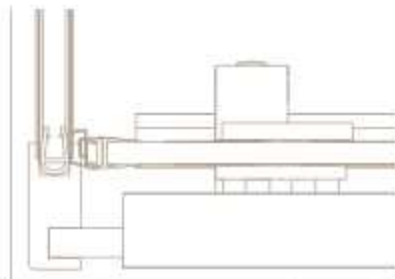
Cierre magnético.
