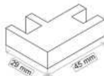
Pieza unión junquillo Acero REF: 039201 20 € REF: 039202 20 €
