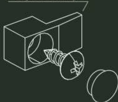
Sujeción cristal fijo
