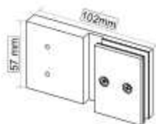
Unión conector - cristal fijo Acero REF: 017801 45 €
