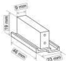
Embellecedor inferior izquierdo conector REF: 012901 10 € ABS
