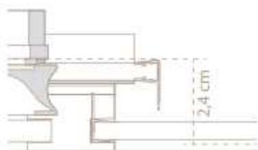
Retranqueo puerta.
