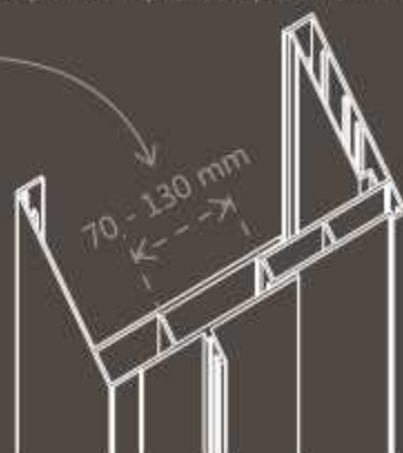
Expansión perfiles para fácil montaje
