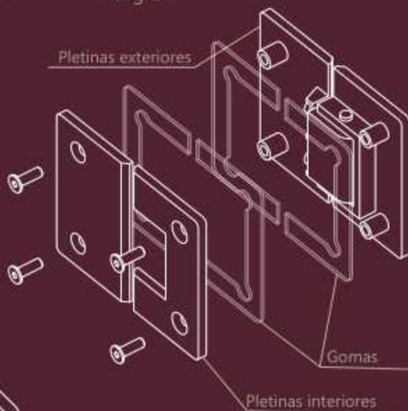
Expansión Pack R
