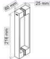
Tirador Acero REF: 024301 44 €
