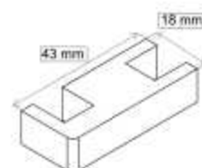
Unión ángulo junquillo Acero REF: 040401 10 € REF: 040402 12 €
