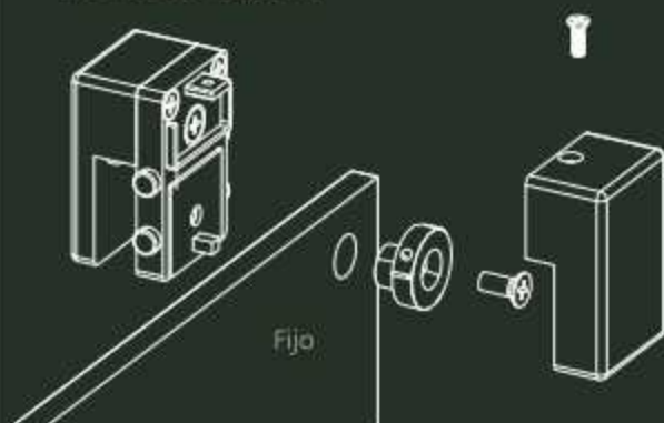
Deslizador superior
