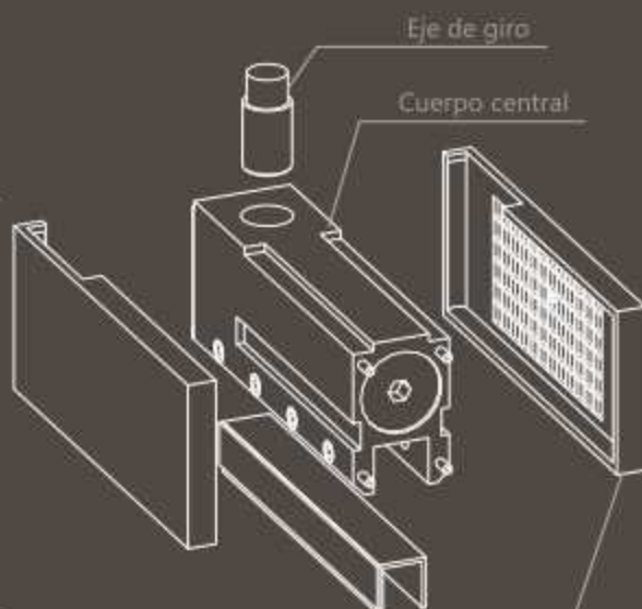
Explosión bisagra superior.
