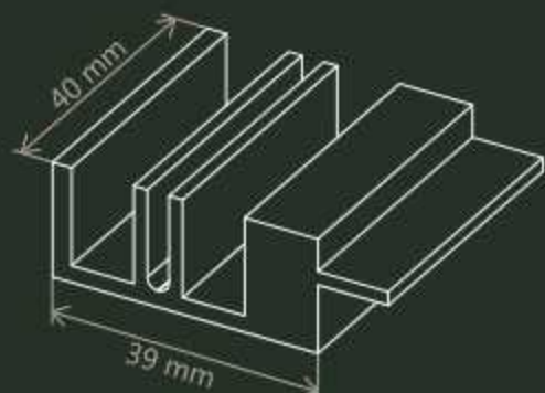
Fijación rail y puerta
