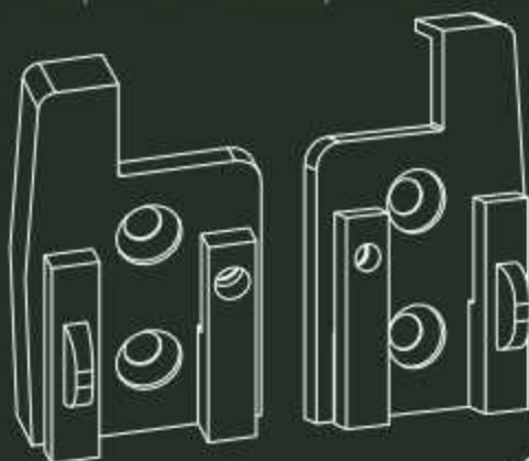
Piezas unión perfil vertical con perfil horizontal
