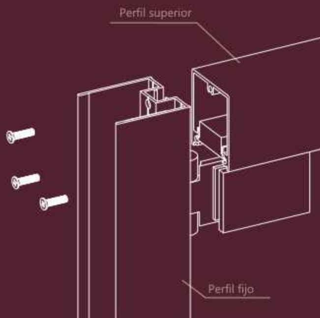
Colocación perfil superior
