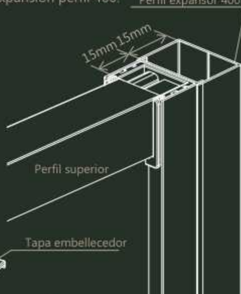
Expansión perfil 400.
