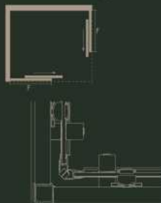
Cierre magnético
