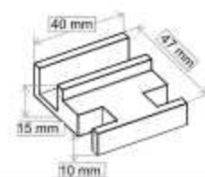
Guiador Acero REF: 038001 25 €
