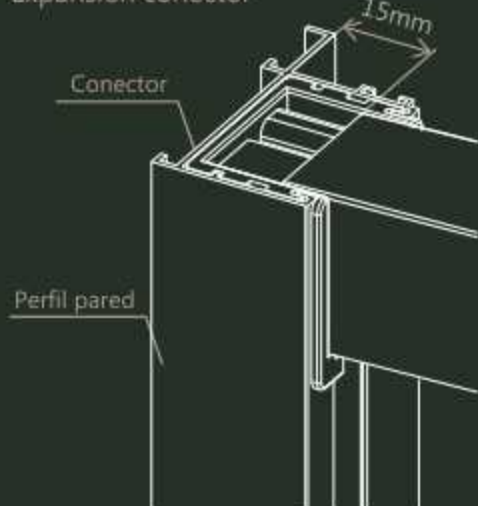
Expansión conector
