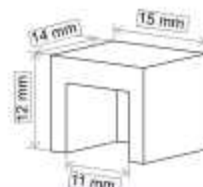
Embellecedor junquillo Acero REF: 040201 10 €
