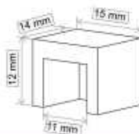
Embellecedor junquillo REF: 040201 10 €
