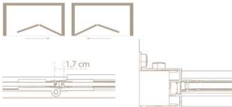
Espacio entre cristales.
