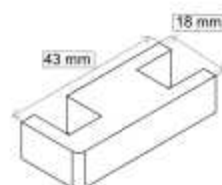
Unión junquillo ángulo Acero REF: 040401 10 € REF: 040402 12 €
