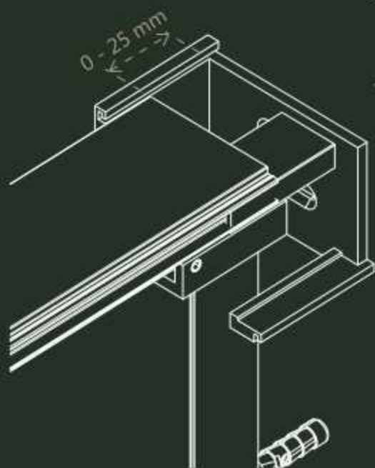
Expansión conector
