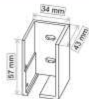
Conector derecha Acero REF: 017701 45 € REF: 017702 50 €
