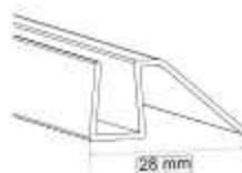
Vierteaguas REF: 035600 11 € Goma
