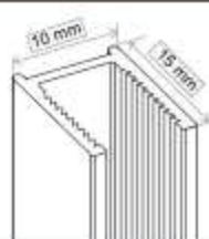
Perfil inferior (opcional) Aluminio REF: 002601 30 € REF: 002602 35 €
