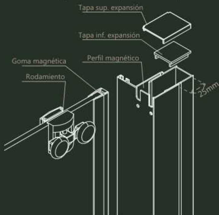
Perfil lateral magnético
