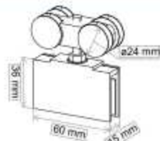
Rodamiento Acero REF: 030401 50 € REF: 030402 60 €
