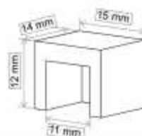
Tapón embellecedor junquillo REF: 040201 10 € Acero
