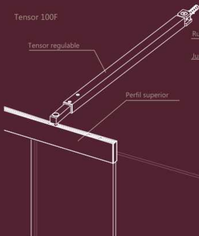
Deslizamiento puerta
