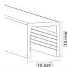
Perfil superior REF: 014301 25 € Aluminio
