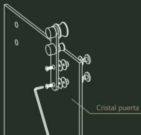
Colocación rodamiento superior
