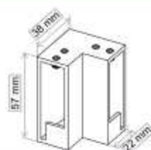
Conector angular perfil superior Acero REF: 013401 45 €
