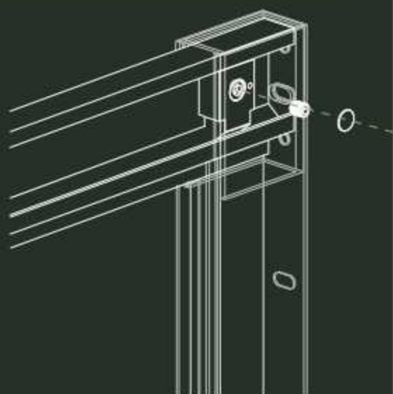
Tirador
