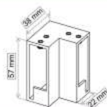
Conector angular perfil superior REF: 013401 45 € Acero
