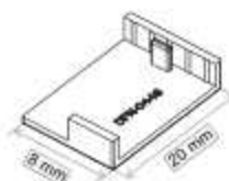
Tapa perfil magnético ABS REF: 005101 10 €
