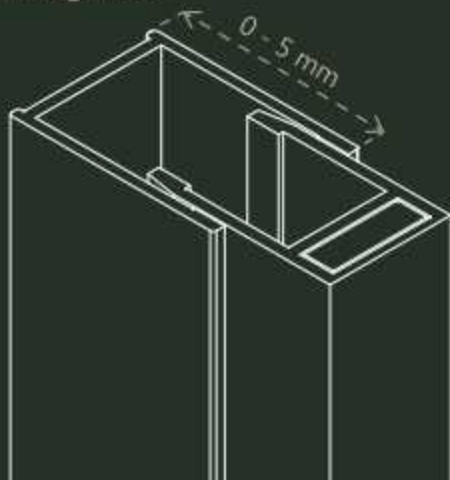
Perfil Magnético
