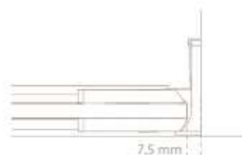
Espacio cristal - pared.
