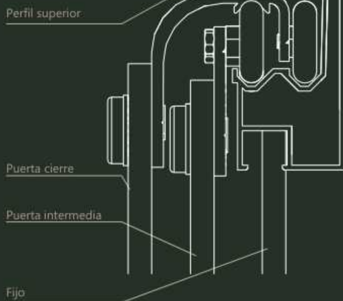
Carril puerta cierre
